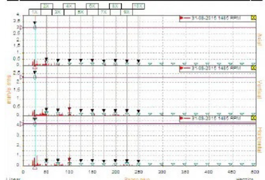
Figura 3. Motor lado acople - Espectro de velocidad
