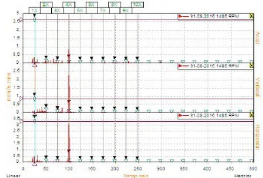
Figura 2. Motor lado opuesto acople - Espectro de velocidad
